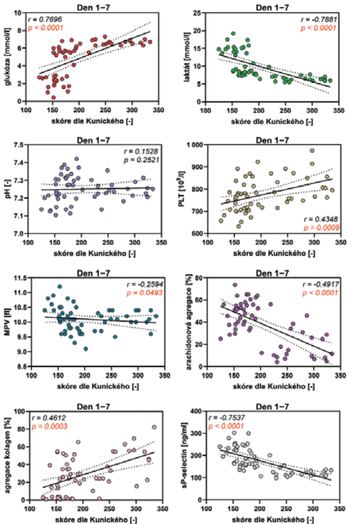
Graf 2. Korelace skóre dle Kunického s dalšími hodnocenými parametry. V grafech je uveden Spearmanův korelační koeficient ( r ) a p -hodnota vyjadřující statistickou signifikanci. V grafech je pro ilustraci dále vynesena jednoduchá lineární regrese s konfidenčními pásy (95%).
