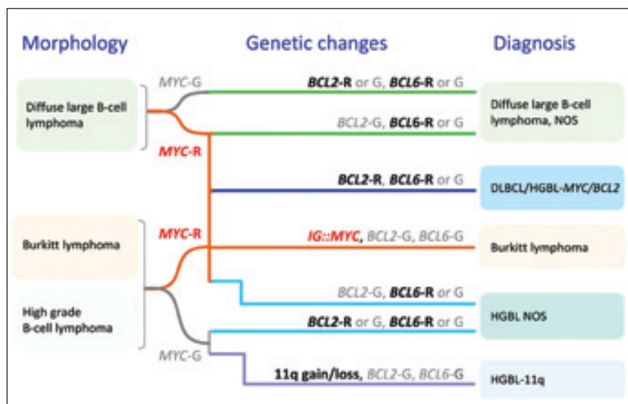
Obr. 4. Algoritmus pro klasifikaci agresivních B-buněčných lymfomů podle WHO-HAEM5. Přestavba genu MYC s jedním s IG genů je diagnostickým kritériem BL, a to na pozadí buněk různé morfologie. Další klasifikační podjednotkou, která je také definována přítomností přestavby genu MYC je DLBCL/HGBL s přestavbou genů MYC a BCL2 . Na rozdíl od BL není přestavba genu MYC spojována s konkrétním translokačním partnerem, kterým může být jak IG gen, tak non-IG partner. Podmínkou pro zařazení této skupiny je současná přítomnost přestavby genu BCL2 , případně přestavby BCL2 i BCL6 . Přestavba genu MYC se může vyskytnout i ve skupinách DLBCL NOS nebo HGBL NOS. Jde o případy přestavby genu MYC s IG i non-IG geny, anebo případy s přestavbou genu MYC a zároveň přestavbou genu BCL6 . Převzato z [34]; užití v souladu s CCL 4.0: https://creativecommons.org/licenses/by/4.0/ ; na obrázku nebyly provedeny žádné změny. R – přestavba; G – germinální uspořádání; IG::MYC – translokace genu MYC k lokusu genu pro imunoglobulinový řetězec; DLBCL, NOS – difúzní velkobuněčný B-lymfom, blíže nespecifikovaný; HGBL, NOS – high-grade B-buněčný lymfom, blíže nespecifikovaný; HGBL-11q – high-grade B-buněčný lymfom s aberacemi 11q.
