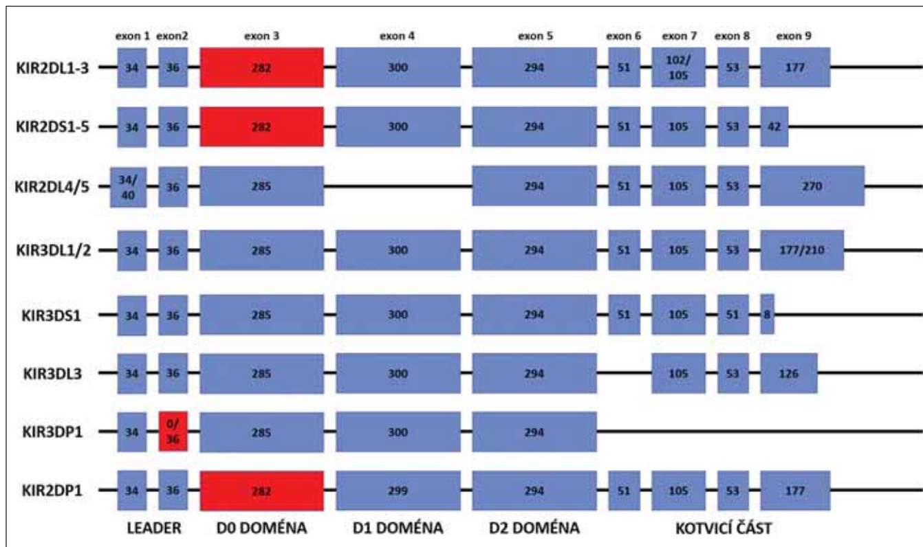
Obr. 1. Struktura genů KIR receptorů, převzato z https://www.ebi.ac.uk/ipd/kir/about/ . Červeně označené jsou pseudoexon 3 a chybějící exon 2 pseudogenu 3DP1. Číslo v boxech značí počet bází. Kotvicí část se skládá ze stonku, transmembránové části a cytoplazmatické části.
