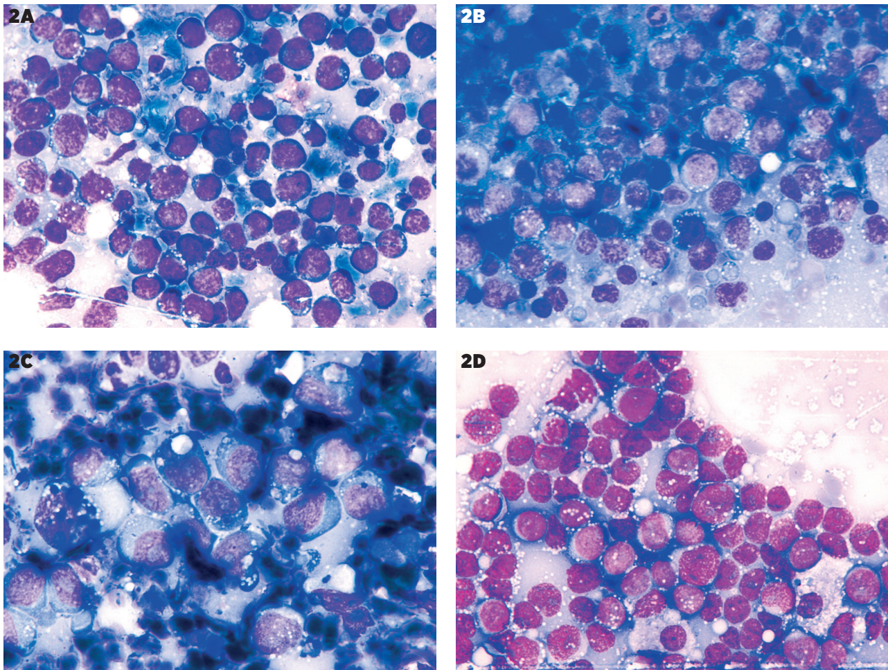
Obr. 2. Infiltrácia bazofilnými vakuolizovanými blastami rôzneho pôvodu Snímky z rovnakého materiálu ako na obrázku 1, zväčšenie 1000x. Blasty alebo blastoidné elementy so silne bazofilnou vakuolizovanou cytoplazmou sa nevyskytujú len pri Burkittovom lymfóme (2A), ale aj pri DLBCL (2B - DLBCL, „triple expressor“) a metastázach: 2C - slabo diferencovaný malígny tumor neurčitého pôvodu a histogenézy, 2D - metastáza melanómu.
