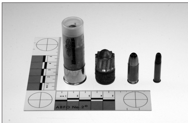
Obr. 1. Struktura náboje Brenneke Classic ráže 16 a typické střely Brenneke stejné ráže ve srovnání s pistolovým nábojem ráže 9 mm Luger a malorážkovým nábojem ráže .22 LR (zleva doprava)
