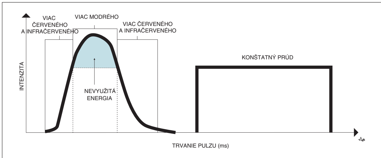
Obr. 1. Porovnanie tvorby pulzu prístrojom s nekontrolovaným vs. kontrolovaným výbojom. V ľavej časti je znázornený priebeh prúdu cez výbojku v prístroji s nekontrolovaným výbojom. Pri postupnom zvyšovaní jeho intenzity je vyžarované spektrum posunuté smerom do červenej a infračervenej časti spektra. V pravej časti je znázornený priebeh prúdu v prístroji s kontrolovaným výbojom. Prúd zostáva počas záblesku konštantný, čím je zaručené vyžiarenie konštantného spektra z výbojky. (Spracované podľa: Town, G., Ash, C., Eadie, E. et al. Measuring key parameters of intense pulsed light (IPL) devices. J Cosmetic Laser Ther , 2007, 9, s. 148 – 160.)
