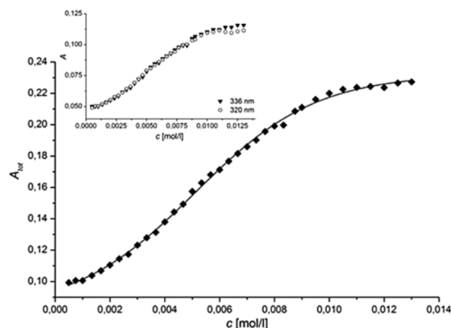
Graf 4. Závislosť súčtu absorpcií hlavných pyrénových píkov ( A_{\text{tot}} ) od koncentrácie ( c ) látky H + B vo vodnom prostredí pri 25 °C
