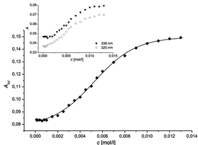
Graf 3. Závislosť súčtu absorpcií hlavných pyrénových píkov ( A_{\text{tot}} ) od koncentrácie ( c ) látky H + Al vo vodnom prostredí pri 25 °C
