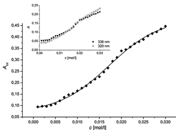
Graf 2. Závislosť súčtu absorpcií hlavných pyrénových píkov ( A_{\text{tot}} ) od koncentrácie ( c ) látky H22 vo vodnom prostredí pri 25 °C
