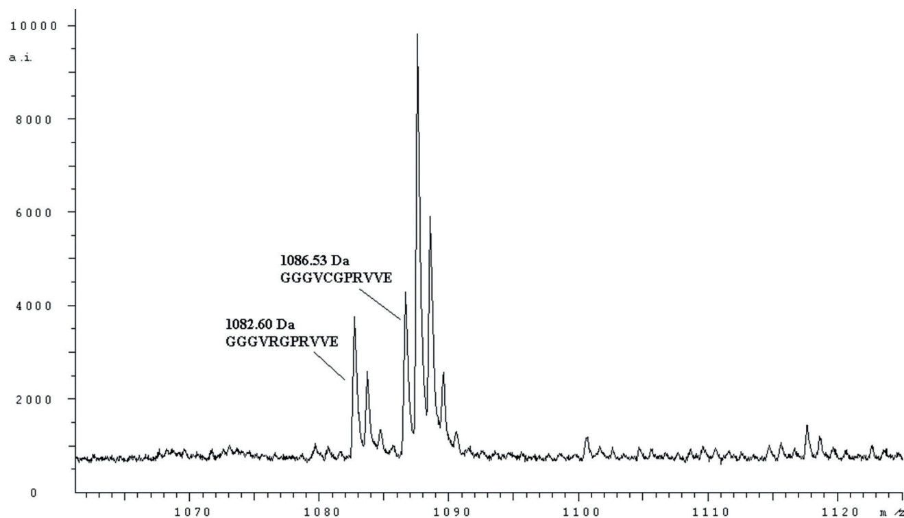
Obr. 1. MH^+ spektrum peptidů fibrinogenu Nový Jičín (štěpeno endopeptidasou Glu-C) odpovídající sekvenci A\alpha 12 – 22. Jsou zobrazeny píky normálního (1082,60 Da, GGGVRGPRVVE) a abnormálního S-karboxamidometylovaného (1086,53 Da, GGGVCGPRVVE) peptidu.
