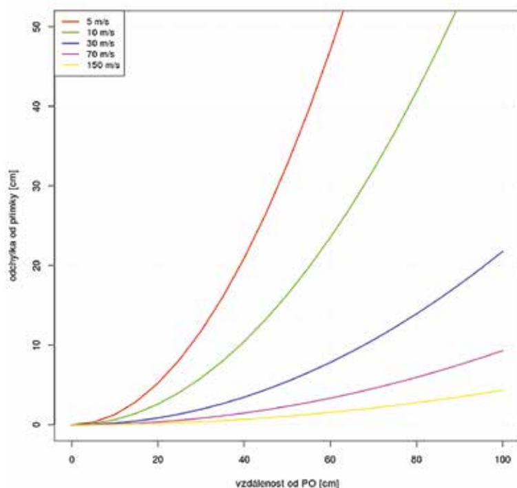
Obr. 1. Odchylna trajektorií modelovaných přímkou a parabolou. Na vodorovné ose je vzdálenost od PO, na svislé ose je vzdálenost trajektorií, vyznačeny jsou křivky pro různé rychlosti letu krevní kapky. S rostoucí rychlostí je zřejmé, že odchylna klesá. Graf byl vytvořen v pomoci jazyka R (ver. 3.2.3).
