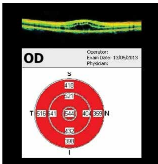
Obr. 9 OCT makuly OP 3 týdny po aplikaci bevacizumabu Ve fovee OP 544 \mu\text{m} , minimální reakce na bevacizumab
