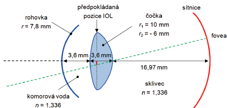
Obr. 5. Gullstrandův zjednodušený schematický model oka
